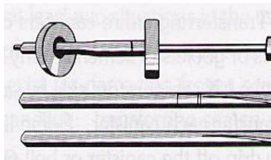
Hình 42: Súng dẫn tinh kiểu vòng nhẫn
